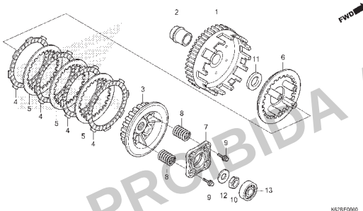
M-8 Embreagem
