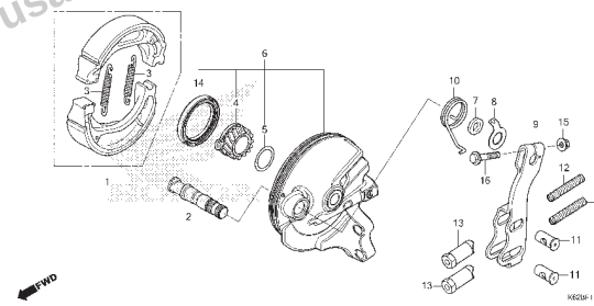
C-13 Painel do Freio Dianteiro
