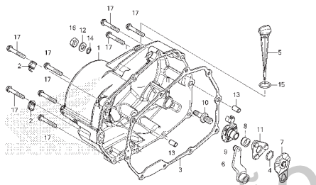
M-9 Embreagem de Partida
