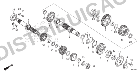
M-17 Transmissão
