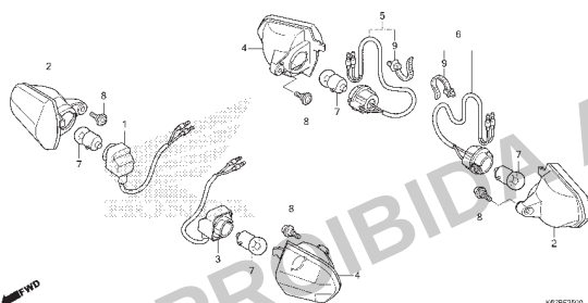
C-35 Sinalizador
