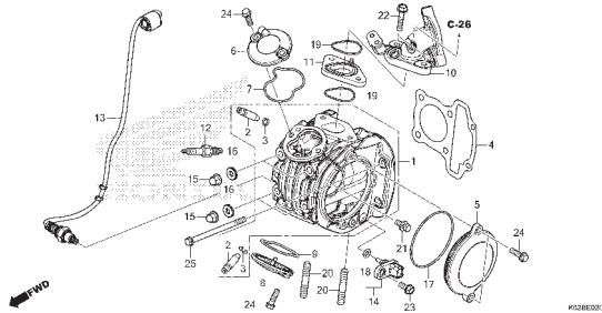
M-5 Cilindro
