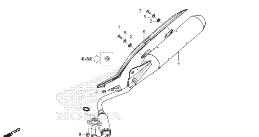
C-27 Escapamento
