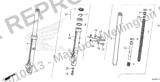
C-11 Garfo Dianteiro
