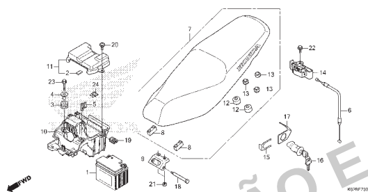
C-26 Câister
